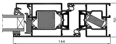
przekrój drzwi
