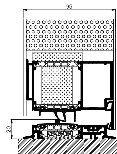
przekrój przez próg drzwi panelowych MB-104 PASSIVE Aero
