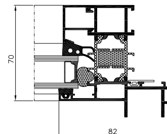
przekrój przez okno MB-70US
