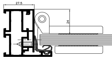
przekrój boczny drzwi
