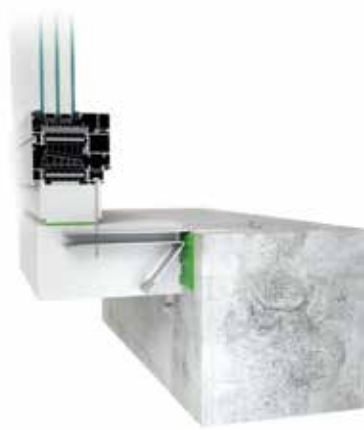
połączenie dolne, na belce 200 mm z kotwą wewnętrzną
