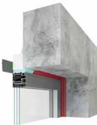
połączenie górne, z taśmą paroszczelną i klejem-uszczelniaczem
