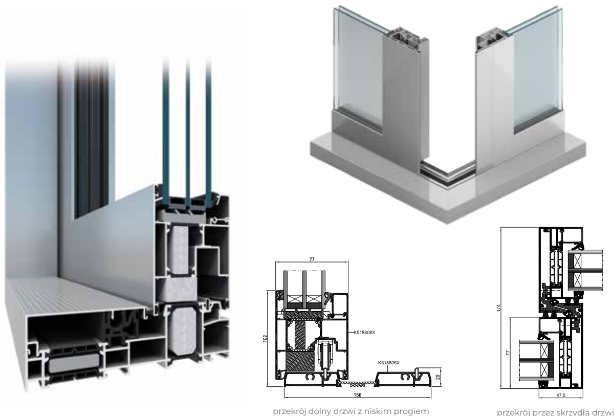
przekrój dolny drzwi z niskim progim
