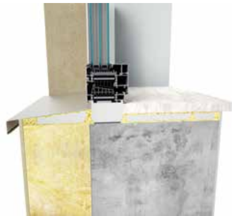
przekrój przez okno zamontowane w licu ściany
