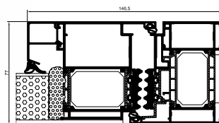
przekrój przez drzwi panelowe MB-86N SI+ w zabudowie witrażowej
