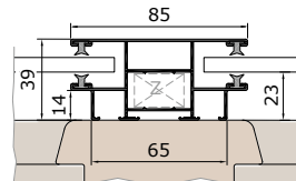
Podpora z prowadnicą KF85V
