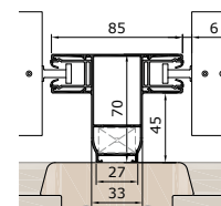
Podpora z ED85V
