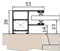
Prowadnica KE53V w przypadku remontu
