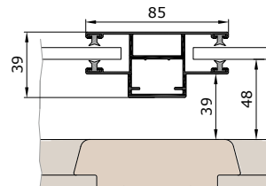
Podpora z prowadnicą samonośną
