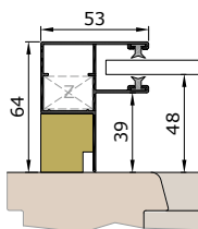
Prowadnica odrębna termicznie KD53VT
