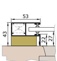
Prowadnica odrębna termicznie K53VT
