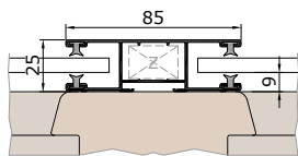
Podpora z prowadnicą K85V
