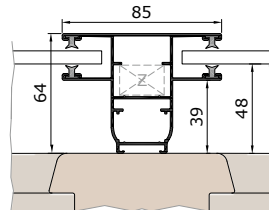
Podpora z prowadnicą KD85V
