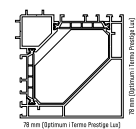
Rysunek techniczny
